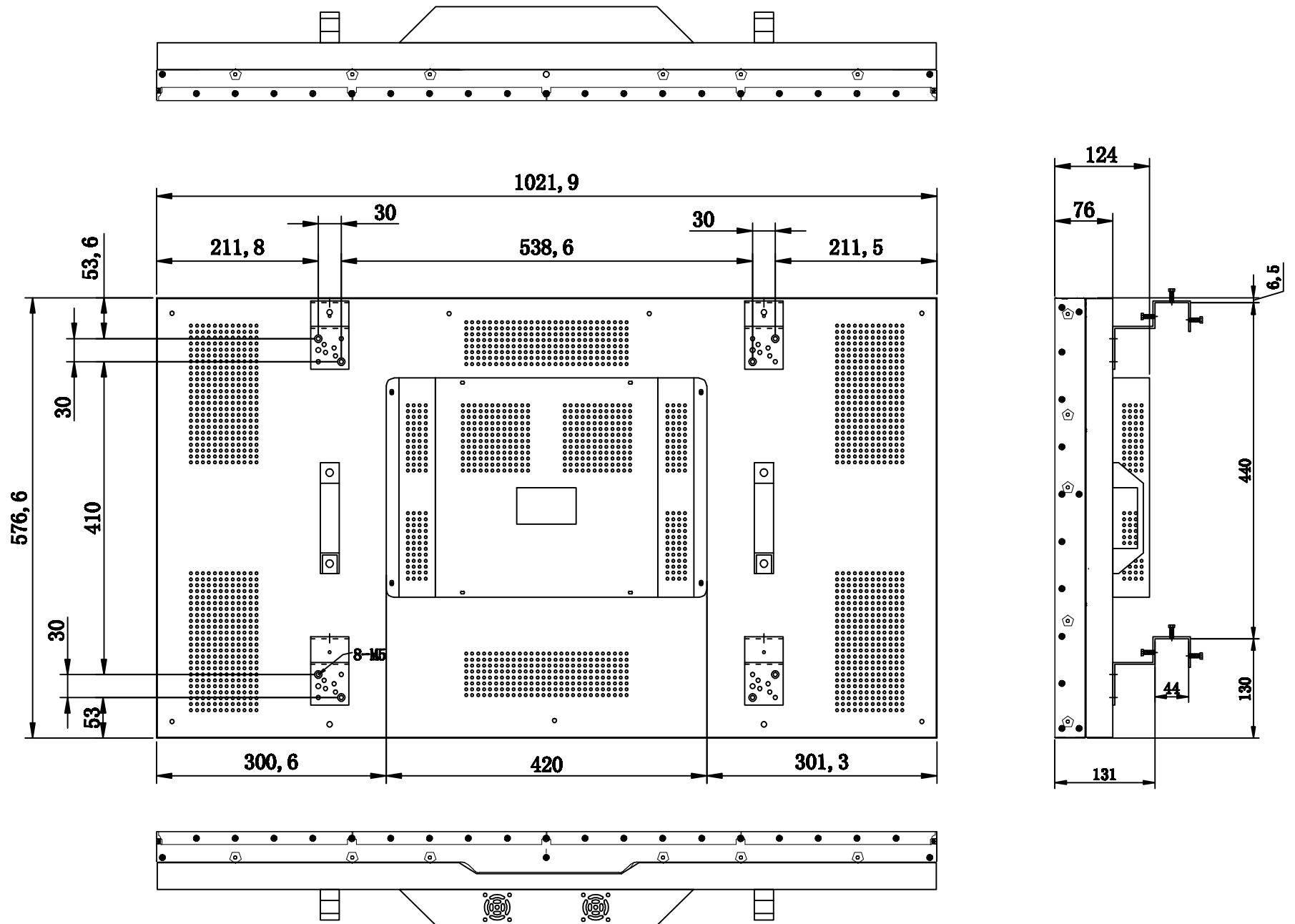
46寸整机图(适用型号: LTI460HN10/LTI460HN11/LTI460HN12)
